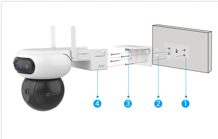
그림 2 벽 장착
